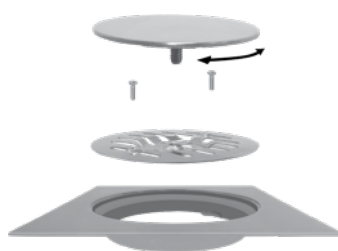
Esploso dei componenti
