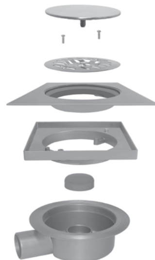
Esploso dei componenti
