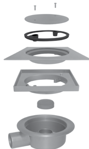
Esplso dei componenti
