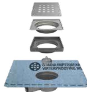
Esploso dei componenti
